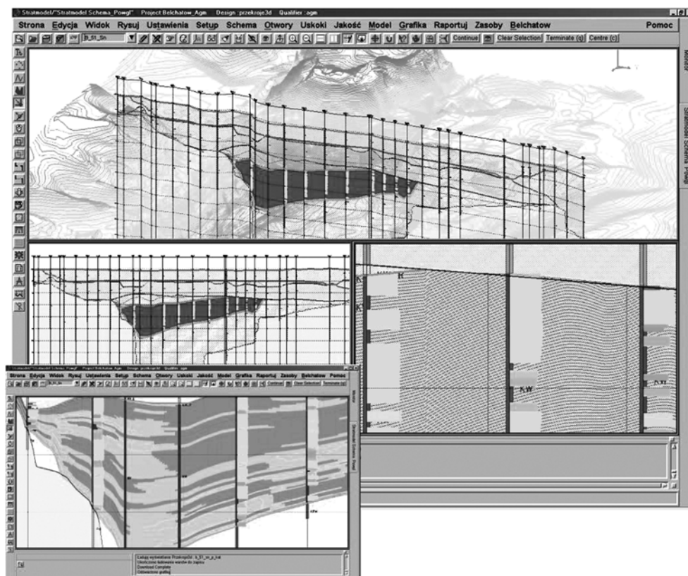
Rys. 9. Struktura modelu plastrowego i kategorie jakościowe oznaczone barwnie na przekroju przez plastry
