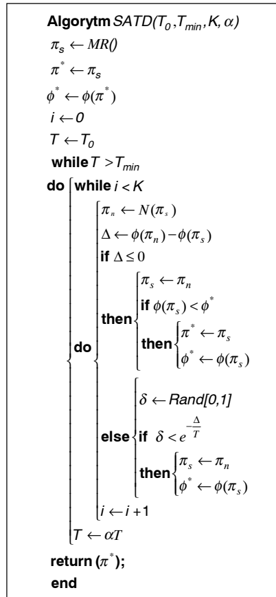
Rys. 2. Algorytm symulowanego wyżarzania SATD dla zagadnienia trójwymiarowego pakowania gdzie:
