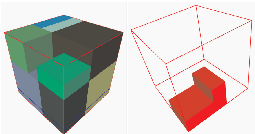
Rys. 3. Przykład pakowania za pomocą algorytmu SATD kontenera 5 \times 5 \times 5 dla n = 125 paczek uzyskanych poprzez ich losową generację rozkładem normalnym ( \mu = 3 , \sigma^2 = 2 ). Współczynnik wypełnienia \phi(\pi^*) = 93\% (z prawej – paczki, z lewej – niewykorzystane miejsce w kontenerze)
