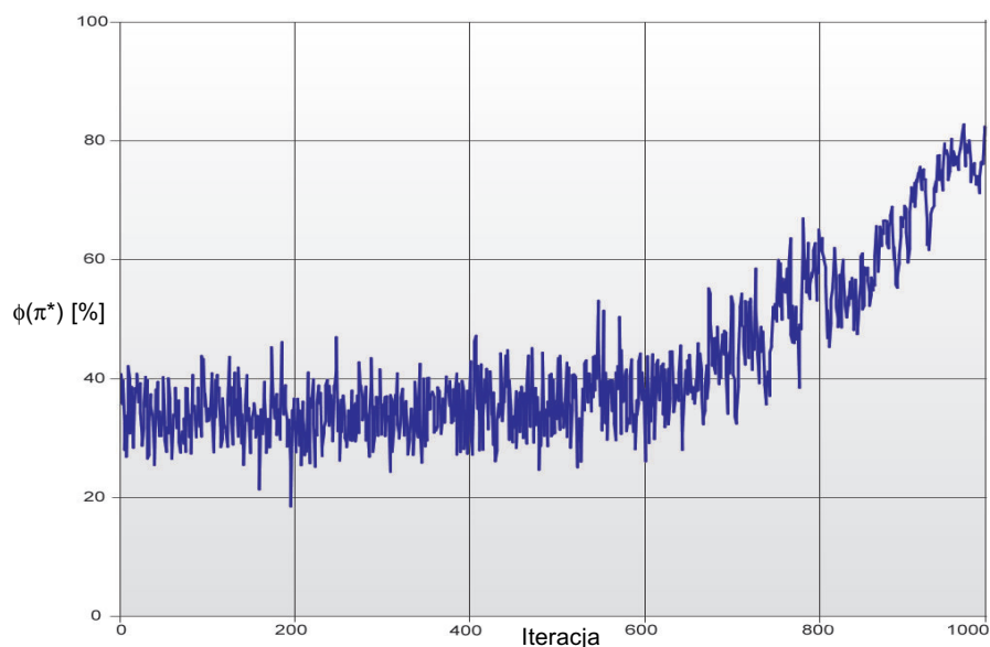
Rys. 4. Ilustracja procesu szukania najlepszego upakowania za pomocą algorytmu SATD kontenera 5 \times 5 \times 5 dla n = 125
