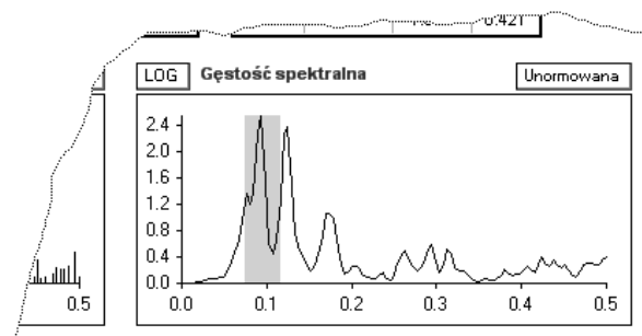
Fig. 7. Program TRIFOUR : Pasma częstotliwości zaznaczone na wykresie funkcji gęstości spektralnej
