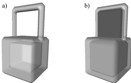
Rys. 6. Wizualizacja półprzezroczystej izopowierzchni obiektu zawierającego jeden otwór i jedną pustkę. Pustka znajduje się wewnątrz sześcianu (a). Wynik zastosowania AZO (ciemny odcień szarości) nałożony na obiekt wejściowy (jasny odcień szarości). Widać, że AZO nie tylko zamknął otwór, ale także wypełnił pustkę (b)
