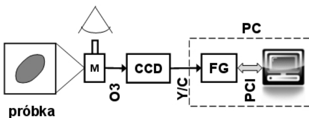
Rys. 1. Schemat blokowy stanowiska pomiarowego. M – mikroskop optyczny, O3 –trinkular, CCD – kamera CCD z interfejsem Y/C, FG – karta akwizycji obrazu, PC – komputer z oprogramowaniem
