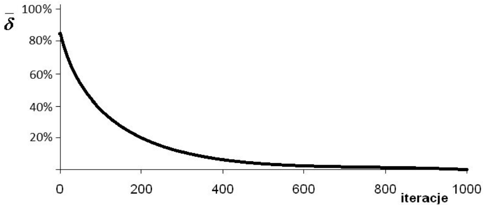
Rys. 3. Zależność średniego błędu rozwiązań algorytmu CSTTS w zależności od wykonanych iteracji dla ustawień restart = 400 , eLT = 0 , sLT = 10
