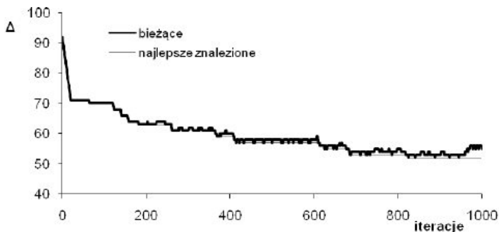
Rys. 2. Przebieg algorytmu CSTTS dla jednego przykładu z 10 grupy, wystawienie algorytmu: liczba iteracji = 1000, restart = 400, eLT = 20 , sLT = 0
