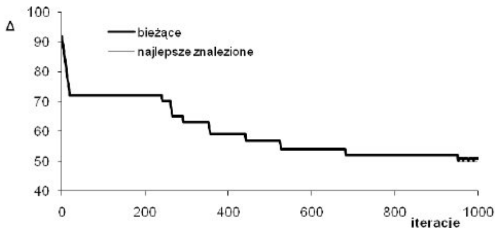
Rys. 1. Przebieg algorytmu CSTTS dla jednego przykładu z 10 grupy, wystawienie algorytmu: liczba iteracji = 1000, restart = 400, eLT = 0 , sLT = 10
