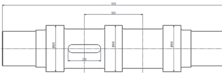
Rys. 4. Przykład osi kół dwulinowych
