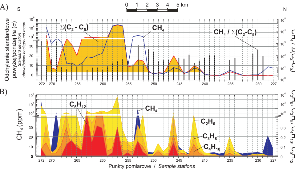
Fig. 7. Zmiany stężeń alkanów wzdłuż profilu F-F: A) wartości znormalizowane i przefiltrowane; B) wartości pomierzone (surowe) Fig. 7. Changes of alkanes concentrations along F-F profile: A) normalized and filtered values; B) raw values
