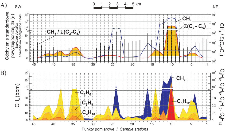
Fig. 6. Zmiany stężeń alkanów wzdłuż profilu A-A: A) wartości znormalizowane i przefiltrowane; B) wartości pomierzone (surowe) Fig. 6. Changes of alkanes concentrations along A-A profile: A) normalized and filtered values; B) raw values
