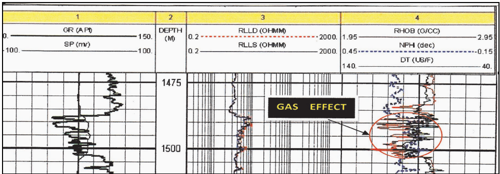
Fig. 8. Composite log
