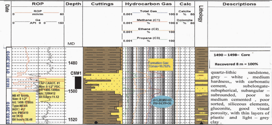
Fig. 6. Litholog
