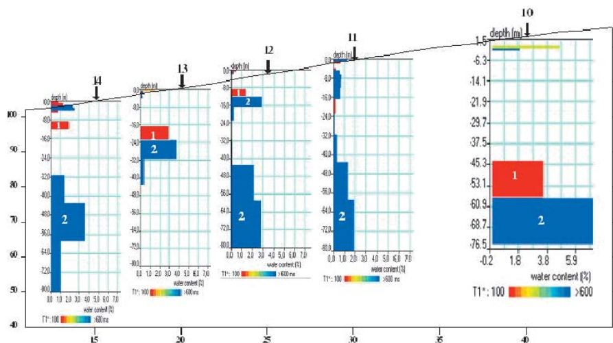
Fig. 4. Results of interpretation for profile T1 by Magnetic Resonance Sounding data in Bac Binh area (1 – fine sand layer, 2 – coarse sand layer) Fig. 4. Wyniki interpretacji sondowań magnetycznego rezonansu jądrowego na obszarze Bac Binh (1 – warstwa piasków drobnoziarnistych, 2 – warstwa piasków różnoziarnistych)
