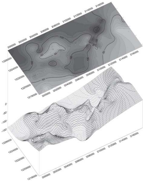
Fig. 6. The structure map of basement (bedrock) for study area on the basis of complex geophysical data Fig. 6. Mapa strukturalna podłoża na obszarze badań wykonana na podstawie wyników kompleksowych badań geofizycznych
