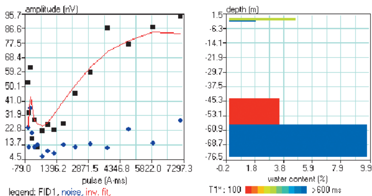
Fig. 3. Result of interpretation of MRS at point 10 – profile T1 in Bac Binh area Fig. 3. Wynik interpretacji sondowania magnetycznego rezonansu jądrowego w punkcie 10 na profilu T1 na obszarze Bac Binh
