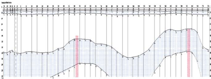
Fig. 5. Section of geological structure of profile TEM (0÷1750 m) by transient EM sounding data (two shadowed layers indicate aquifers) Fig. 5. Przekrój geologiczny wzdłuż profilu TEM (0÷1750 m); sondowania elektromagnetyczne (dwie szare warstwy oznaczają dwa poziomy wodonośne)
