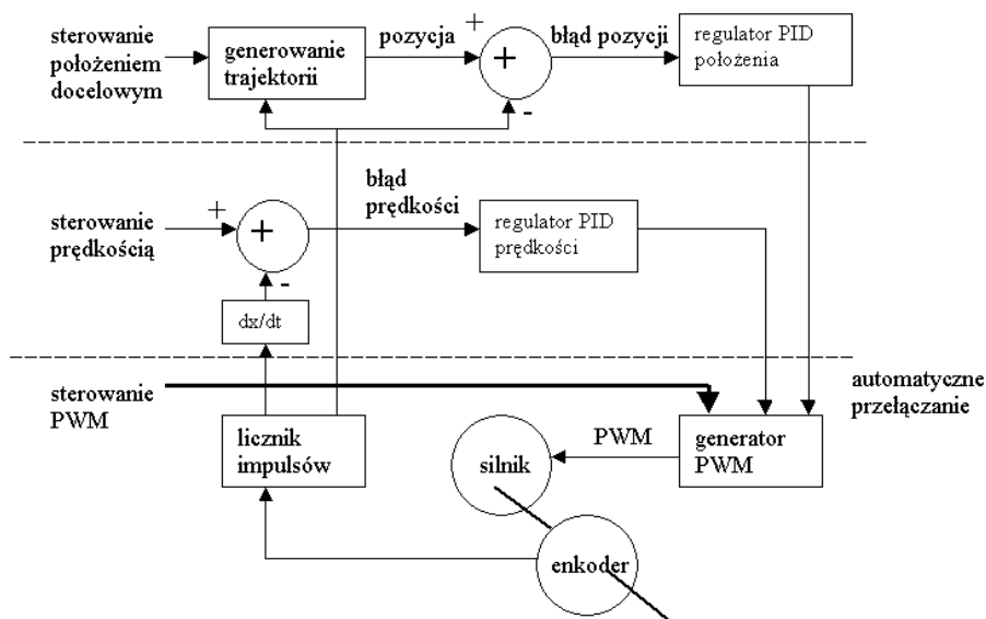
Rys. 5. Schemat sterownika
