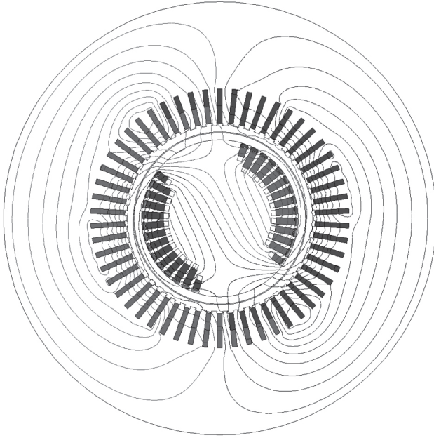
Rys. 4. Rozkład pola magnetycznego oraz gęstości prądów w stanie zwarcia udarowego
