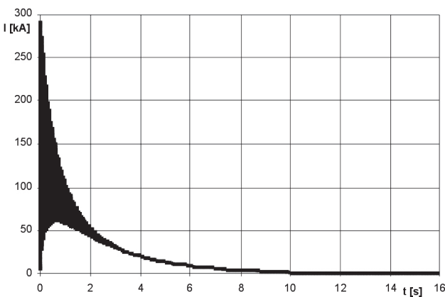
Rys. 6. Składowe nieustalone w prądzie fazowym
