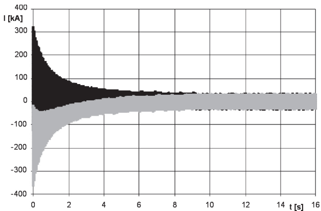
Rys. 5. Prądy fazowe podczas zwarcia udarowego
