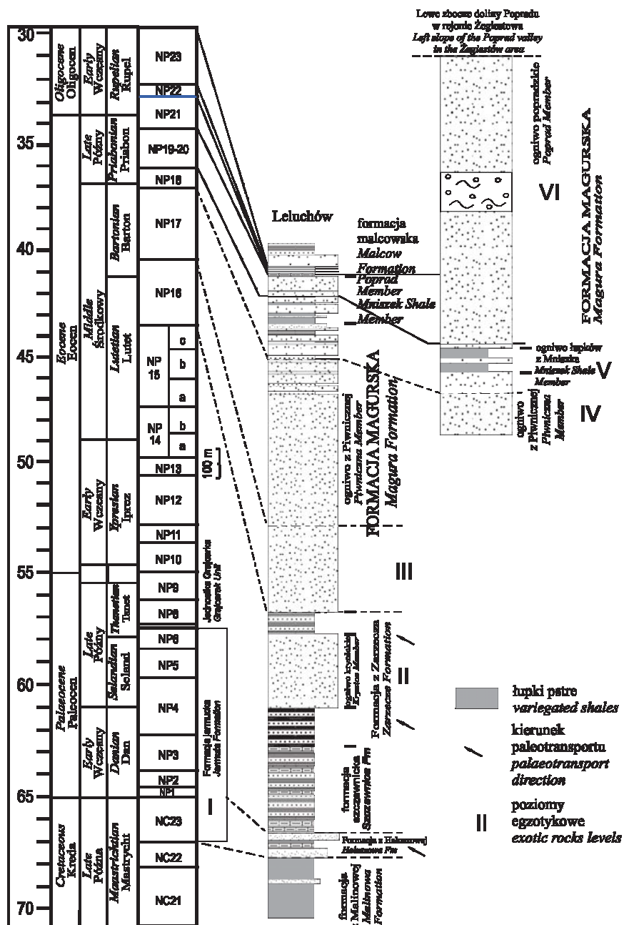
Fig. 2. Profil litostratygraficzny strefy krynickiej płaszczowiny magurskiej (wg Oszczypko-Clowes 2001, uzupełniony)
