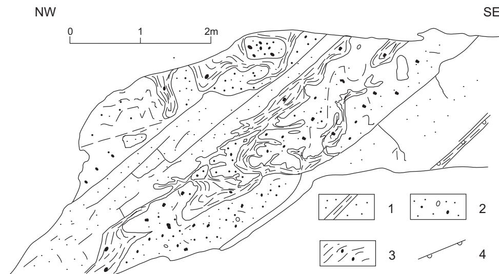
Fig. 3. Szkic odsłonięcia osuwiskowej serii egzotykowej w Przysietnicy (ogniwo piaskowców krynickich formacji zarzeczkiej, wg Oszczypko 1975, uzupełniony): 1 – piaskowce gruboławicowe z przeławiczeniami łupków ilastych, 2 – parzlepnięcia egzotykowe, 3 – żwirowce ilaste, 4 – położenie spągu warstw
