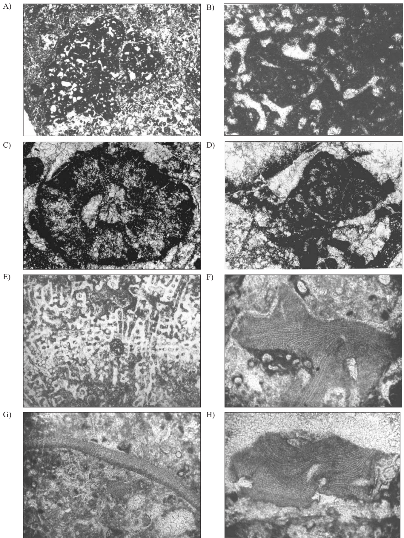
Fig. 7. A)–D) mikrofakcja wapieni urgońskich (barrem-apt) (A, D – Zarzecze; B, C – Kadcza); E)–H) wapień litotamniowo-koralowcowe (paleocen?) – Kadcza; A) pow. 12×, B) pow. 35×, C) pow. 42×, D) pow. 35×, E) pow. 20×, F)–G) pow. 57× (Oszczypko 1975)
