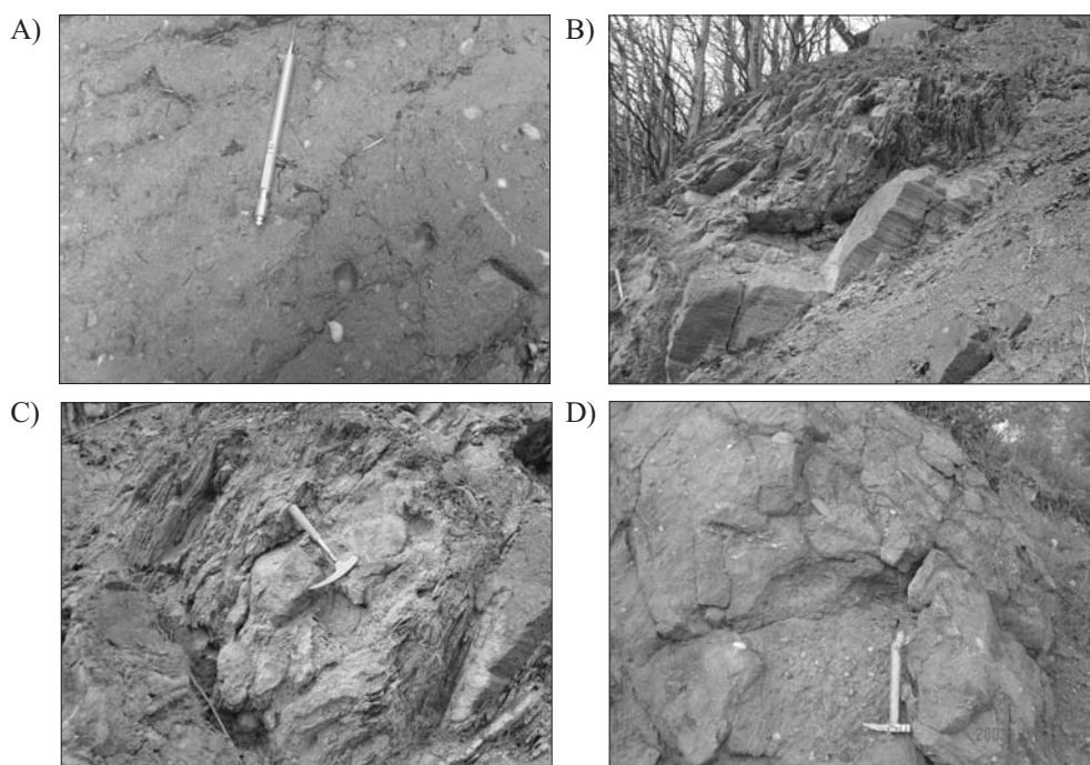
Fig. 5. Fotografie odsłonieć egzotycznych: A) żwirowce ilaste, potok Wilcze k. Muszyny (ogniwo piaskowców krynickich formacji zarzeczkiej); B) osuwiskowa seria egzotyczna w Piwnicznej (wyższa część ogniwa piaskowców z Piwnicznej formacji magurskiej); C) jak wyżej, szczegół serii osuwiskowej; D) egzotyczny żwirowiec ilasty w Leluchowie (wyższa część ogniwa piaskowców z Piwnicznej formacji magurskiej)
