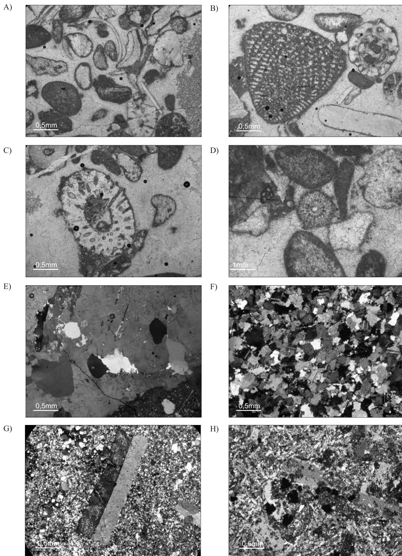
Fig. 8. A)–D) mikrofacja wapieni urgońskich (apt) (Leluchów); E) granitoid (Zarzeczce); F) aplit (Zarzeczce); G) skała typu ryolitu (Zarzeczce); H) skała typu trachitu (?) (Zarzeczce); fot. A)–D) 1 nikol; fot. E)–H) X nikole
