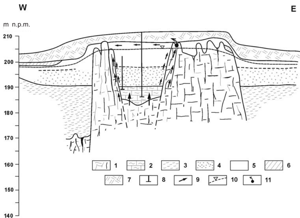
Fig. 3. Schematyczny przekrój hydrogeologiczny rejonu Starego Miasta w Krakowie: 1 – wapień jurajskie, 2 – margle kredowe, 3 – iły miocenijskie, 4 – żwiry i piaski czwartorzędowe, 5 – piaski czwartorzędowe, 6 – torfy czwartorzędowe, 7 – nasypy antropogeniczne, 8 – otwory wiertnicze, 9 – kierunki przepływu wód podziemnych, 10 – zwierciadło wód podziemnych, 11 – stare źródło solanki na Rynku Głównym
