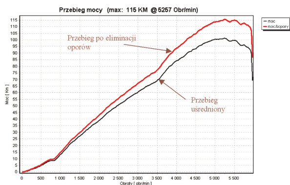
Rys. 17. Wynik uśrednień oraz działania algorytmu eliminacji oporów dla przebiegu mocy
