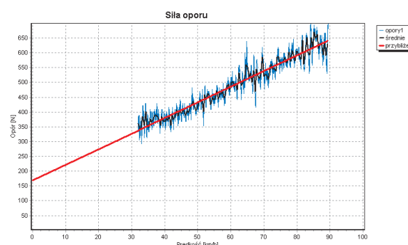
Rys. 15. Zależność siły oporu działającej na samochód w zależności od prędkości oraz przybliżenie prostą
