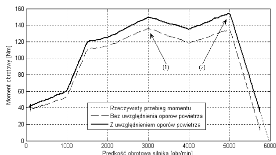
Rys. 10. Wykres momentu obrotowego otrzymany w wyniku pomiaru. (1), (2) – Wartości maksymalne przebiegów
