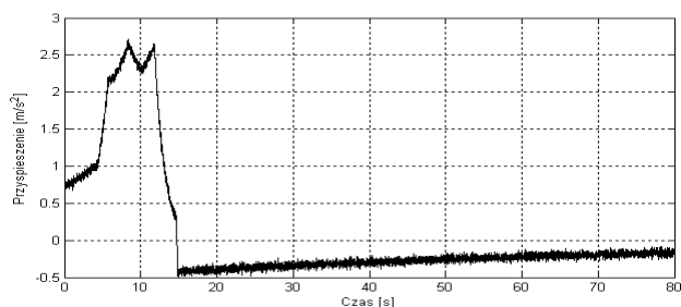
Rys. 8. Przyspieszenie pojazdu zarejestrowane w czasie symulacji
