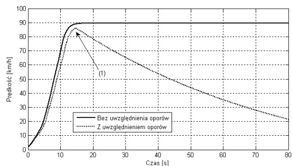
Rys. 7. Przebieg prędkości samochodu w czasie symulacji
