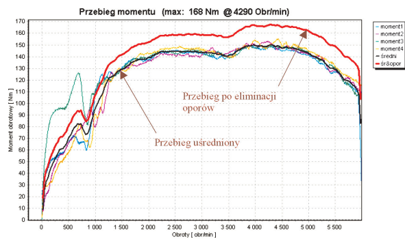
Rys. 16. Wynik uśrednień oraz działania algorytmu eliminacji oporów dla przebiegu momentu obrotowego
