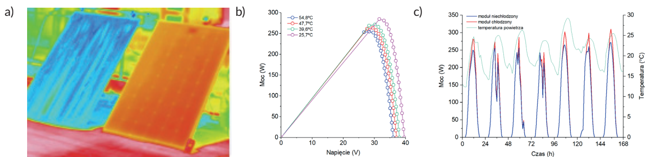
Rys. 20. Prototyp systemu wodnego chłodzenia i czyszczenia modułów PV: a) termogram ilustrujący różnicę w temperaturze powierzchni modułu niechłodzonego i chłodzonego; b) charakterystyki pracy testowanego modułu; c) przebieg zmian mocy generowanej w niechłodzonym i chłodzonym module fotowoltaicznym oraz temperatury powietrza zewnętrznego w wybranym tygodniu lipca
