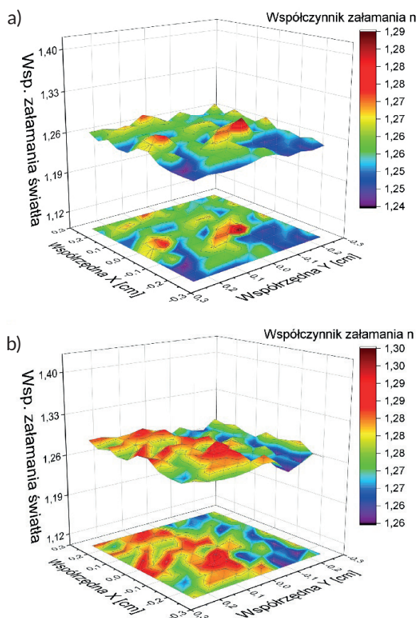
Rys. 13. Mapy jednorodności współczynnika załamania światła n : a) przed napromieniowaniem; b) po napromieniowaniu protonami o energii 226,5 MeV
