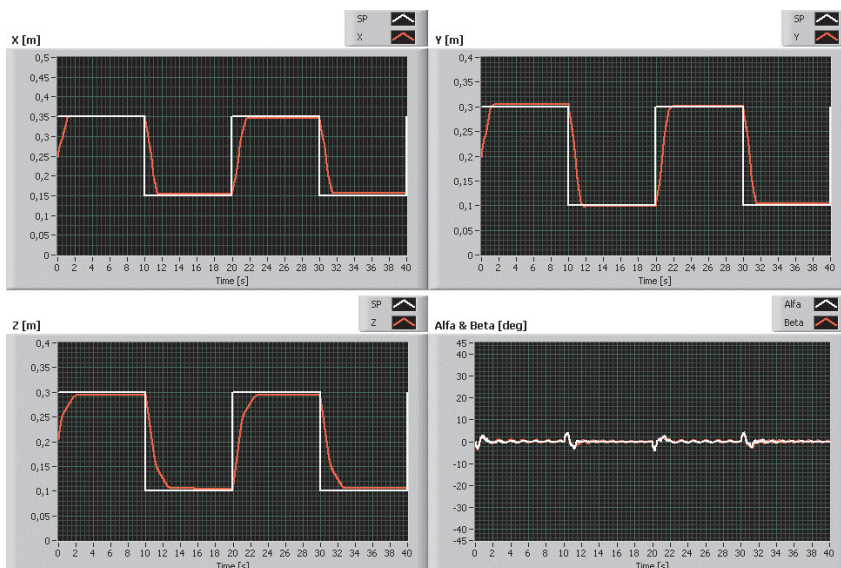
Rys. 16. Regulacja (nadążna) położen wózka i mostu i wysokości ciężarka z aktywnym tłumieniem drgań ciężarka
