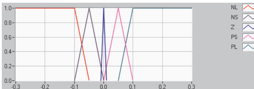
Rys. 4. Graficzna reprezentacja funkcji przynależności dla sygnałów wejściowych (błąd położenia) regulatora typu P – dla kierunków wzdłuż osi x , y i z
