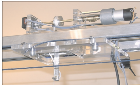
Rys. 2. Wózek z zamontowanym układem do pomiaru kątów wychyleń ciężarka
