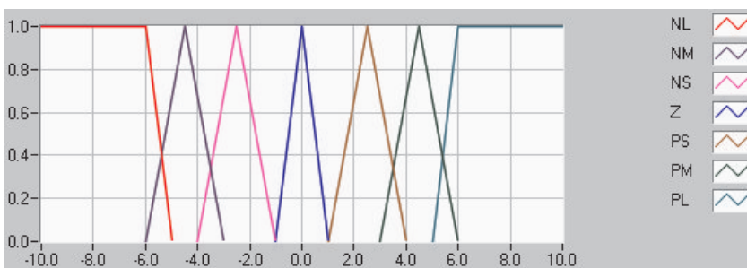
Rys. 7. Graficzna reprezentacja funkcji przynależności dla sygnałów wejściowych (błąd odchylenia kątowego) regulatora typu PD dla kątów \alpha i \beta
