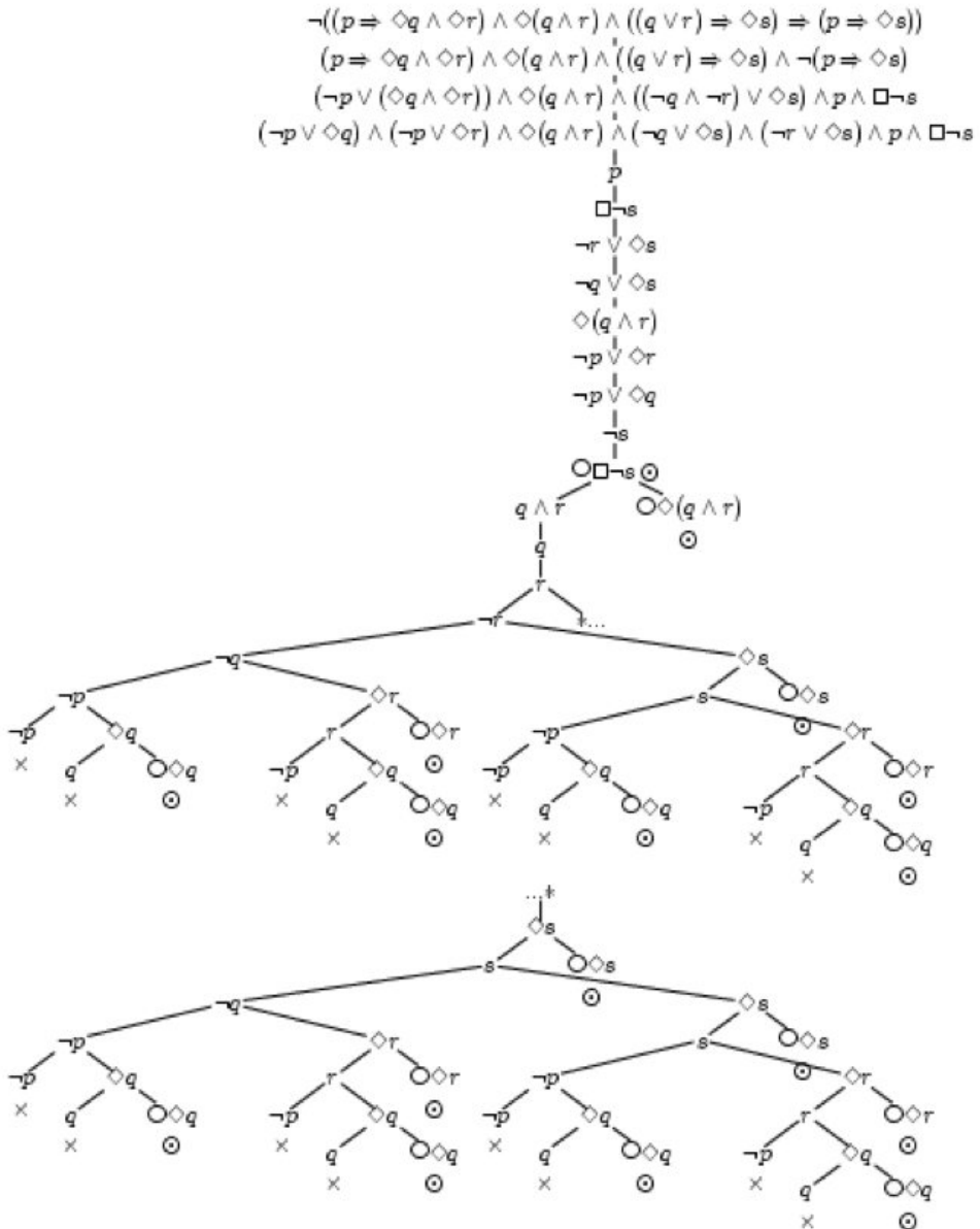
Rys. 3. Drzewo wnioskowania dla rozważanego przypadku
