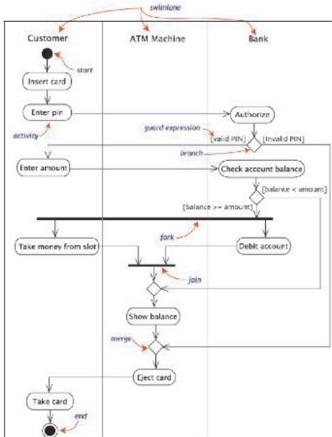
Rys. 1. Przykładowy opis scenariusza przypadku użycia „Pobierz pieniądze z bankomatu” zapisany w formie diagramu czynności
