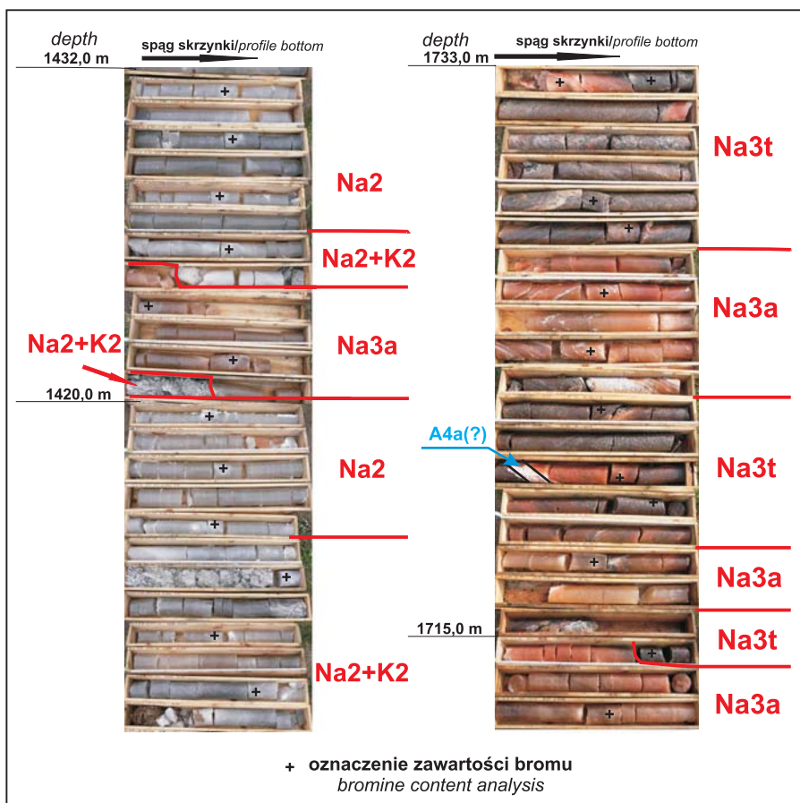
Fig. 3. Fragmenty rdzenia z profilowanego otworu wiertniczego G-34. Objasnienia wydzieliń litrostratygraficznych w tekście jak na figurze 2, Na3a – młodsza sól kamienna dolna, A4a – anhydryt pegmatytowy
