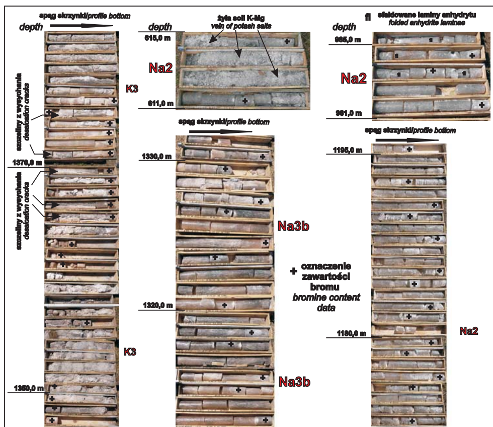
Fig. 4. Fragmenty rdzenia z profilowanych otworów wiertniczych G-16 i G-39. Objasnienia wydzielen litostratygraficznych jak na figurze 2, Na3b – młodsza sól kamienna górna, K3 – młodsza sól potasowa
