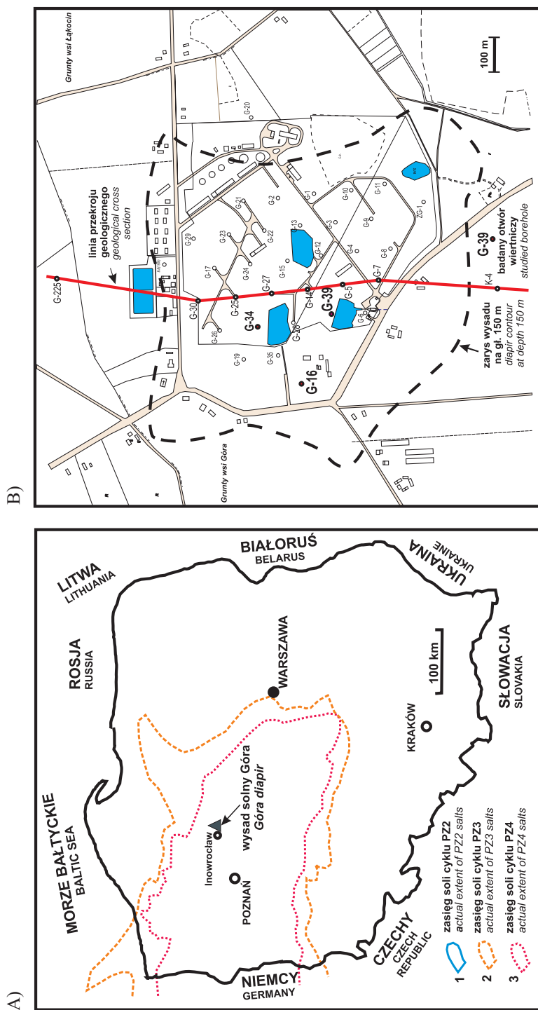
Fig. 1. Lokalizacja badanych otworów wiertniczych na wydzie solnym Góra: A) położenie wydasy Góra na tle aktualnego rozmieszczenia utworów solnych cechszynu w Polsce (wg Czapowskiego 1995); B) rozmieszczenie otworów wiertniczych na terenie wydasy Góra
