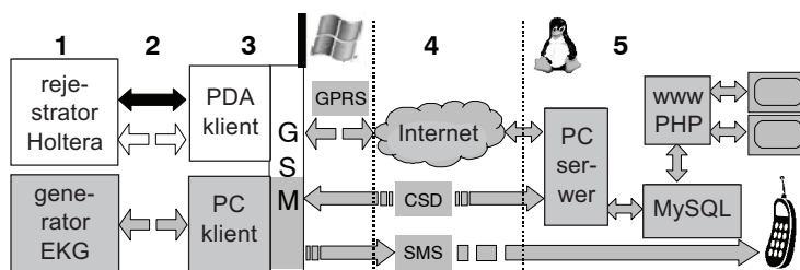
Rys. 2. Oprogramowanie zdalnego nadzoru kardiologicznego. Szarym kolorem oznaczono część zaimplementowaną i przetestowaną. Cyfry odnoszą się do elementów pokazanych na rysunku 1
