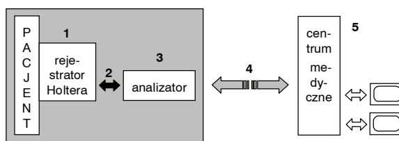
Rys. 1. Schemat systemu zdalnego nadzoru kardiologicznego. Prostokątem w kolorze szarym oznaczono część lokalną – otoczenie pacjenta
