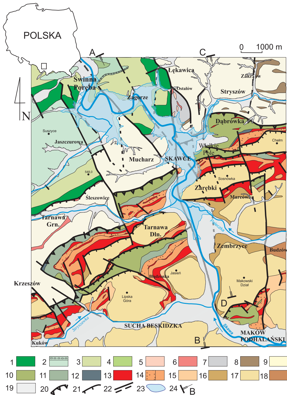
Fig. 1. Mapa geologiczna z elementami tektoniki rejonu na północ od Suchoj Beskidzkiej (wykorzystano materiały z publikacji Książkiewicz 1951a, b, 1974a, b, Golonka et al. 1981). Płaszczowina śląska: 1 – warstwy godulskie środkowe – senon, 2 – warstwy godulskie górne (ze zlepieniem malinowskim) – senon, 3 – warstwy istebniańskie dolne – senon, 4 – warstwy istebniańskie górne – paleocen, 5 – piaskowce ciężkowickie – dolny eocen, 6 – łupki pstre – dolny eocen, 7 – warstwy hieroglifowe – dolny-środkowy eocen, 8 – warstwy menilitowe – dolny oligocen, 9 – warstwy krośnieńskie – oligocen. Płaszczowina magurska: Formacja z Jaworzynki – senon-paleocen: 10 – formacja z Jaworzynki – senon-paleocen, 11 – ogniwo piaskowców z Mutnego – paleocen, 12 – ogniwo łupków z Gołyni – paleocen. Formacja z Łabowej – górny paleocen-środkowy eocen: 13 – pstre łupki formacji z Łabowej – górny paleocen-środkowy eocen, 14 – ogniwo piaskowców z Żurawnicy (z kropkami) – górny paleocen, ogniwo piaskowców ze Skawiec – eocen dolny-środkowy, 15 – formacja beloweska – eocen środkowy-górny. Formacja makowska – górny eocen-oligocen: 16 – ogniwo łupków zembrzyckich – górny eocen, 17 – ogniwo piaskowców z Wątkowej – górny eocen-oligocen, 18 – ogniwo łupków budzowskich – oligocen, 19 – utwory czwartorzędowe, 20 – nasunięcie płaszczowiny magurskiej, 21 – nasunięcia, 22 – uskoki, 23 – zasięg zbiornika wodnego Świnna Poręba, 24 – linie przekrojów
