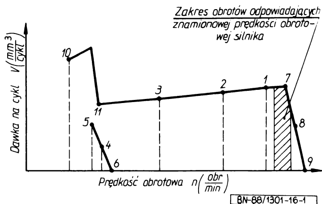
Rys. 1. Przebieg pełnej charakterystyki prędkościowej wydatku pompy wtryskowej
