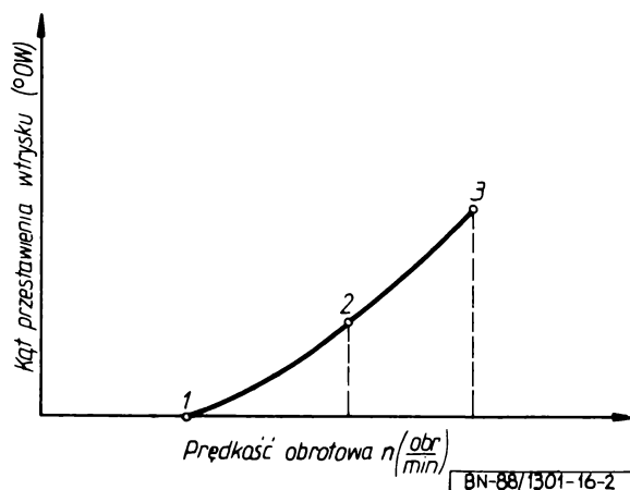
Rys. 2. Przebieg charakterystyki prędkościowej automatycznego przestawiacza wtrysku
