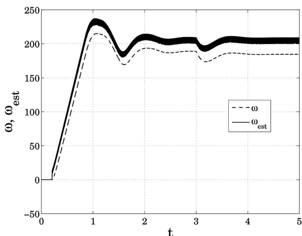
Rys. 10. Porównanie przebiegu prędkości kątowej dla -10% błędu identyfikacji R – wzmocnienie I_1 = 550 ( \max |\psi - \psi_{est}| > 10\% )
