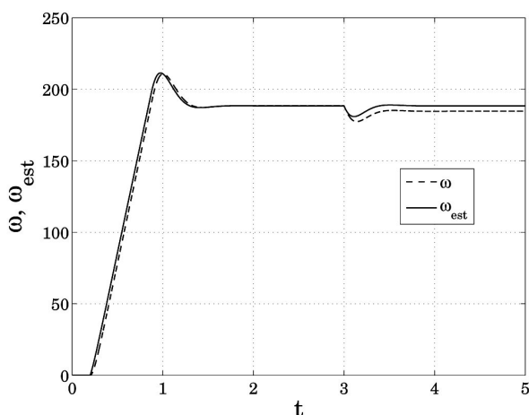
Rys. 11. Porównanie przebiegu prędkości kątowej dla -10% błędu identyfikacji R – wzmocnienie I_1 = 500 ( \max |\psi - \psi_{est}| = 2\% )
