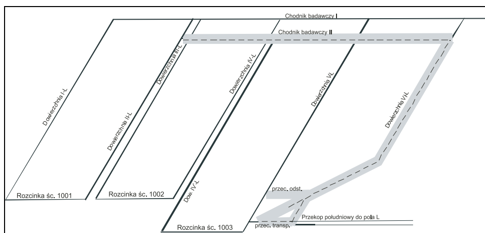
Rys. 3. Warunki hydrogeologiczne w rejonie użytku ekologicznego źródła Kłodnicy
