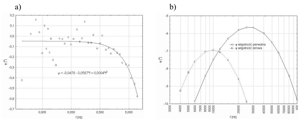
Rys. 4. Zarejestrowane z rysunku 3 fragmenty kąta przesunięcia elektrycznego \varphi odpowiadające maksymalnej wartości tego kąta dla: a) piasku drobnziarnistego; b) bentonitu
