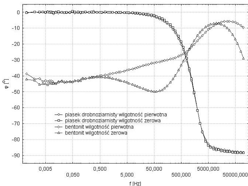
Rys. 3. Zarejestrowane zmiany kąta przesunięcia elektrycznego \varphi piasku drobnziarnistego i bentonitu
