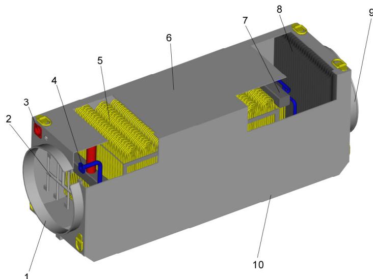
Rys. 2. Parownik chłodziarki powietrza w obudowie: 1 – wlot powietrza, 2 – zraszacz, 3 – króciec ssący, 4 – króciec tłoczący, 5 – węzownica, 6 – obudowa, 7 – kolektor, 8 – wykrapłacz, 9 – wylot powietrza, 10 – płyty transportowe
