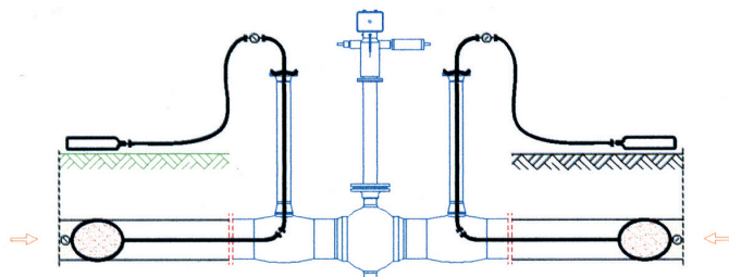
Rys. 12. Dopasowanie nowego ZZU (wraz z naciągnięciem szybkozłączek)
