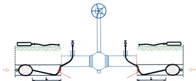
Rys. 7. Wyciąganie ZZU i rozłączenie szybkozłączek (z wyciągnięciem przewodów)
