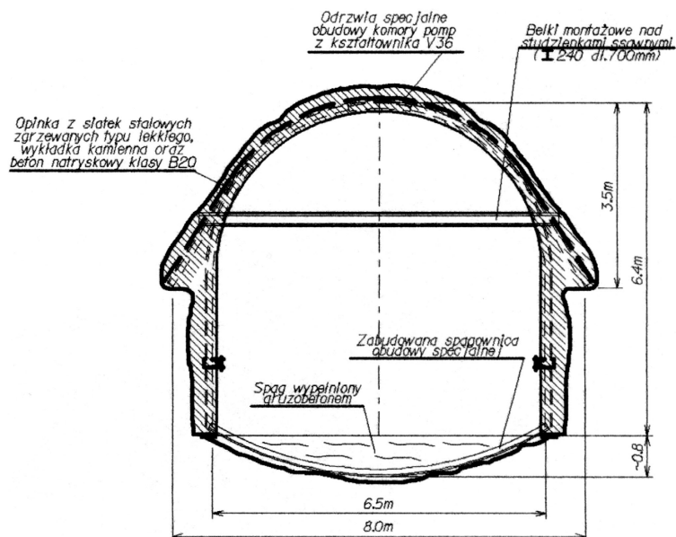
Rys. 6. Odrzvia specjalnej V36 obudowy komory pomp wraz ze spągnicą, zabudowanymi belkami montażowymi oraz wykonanym betonem natryskowym
