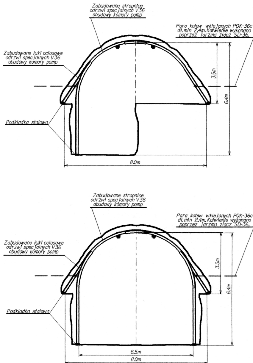
Rys. 4. Zabudowa łuków ociosowych odrzwi specjalnych V36 obudowy komory pomp (kolejne etapy wykonawstwa)
