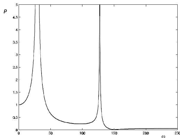
Rys. 7. Współczynnik przenoszenia drgań układu wibroizolacji pokazanego na rysunku 5
