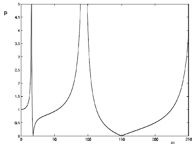
Rys. 4. Współczynnik przenoszenia drgań układu wibroizolacji pokazany na rysunku 2
