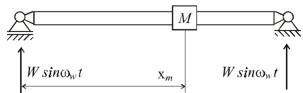
Rys. 5. Model układu wibroizolacji
