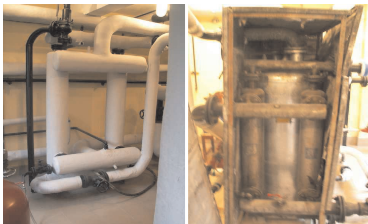
Rys. 2. Wymienniki CO i CWU wraz ze zbiornikiem ciepłej wody w węźle ciepłowniczym jednego z akademików Miasteczka Studenckiego AGH
