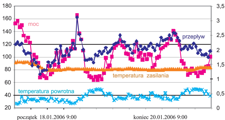
Rys. 8. Dane z wielofunkcyjnego miernika „Controlotron”. Na pionowej osi z lewej strony temperatury odczytywać należy w °C, natomiast moc w kW. Przepływ należy odczytywać z prawej strony w m 3 /h. Na poziomej osi podany jest czas pomiarów
