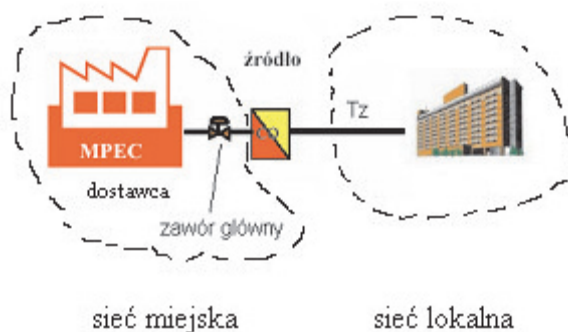
Rys. 4. Schemat dostarczania energii ciepłej do budynku Miasteczka Studenckiego AGH
