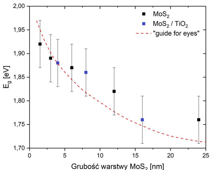
Rysunek 55 Szerokość przerwy energetycznej w funkcji grubości warstwy \text{MoS}_2 dla cienkich warstw \text{MoS}_2 (SERIA 1) oraz heterozłączy planarnych \text{MoS}_2 / \text{TiO}_2 (SERIA 2).
