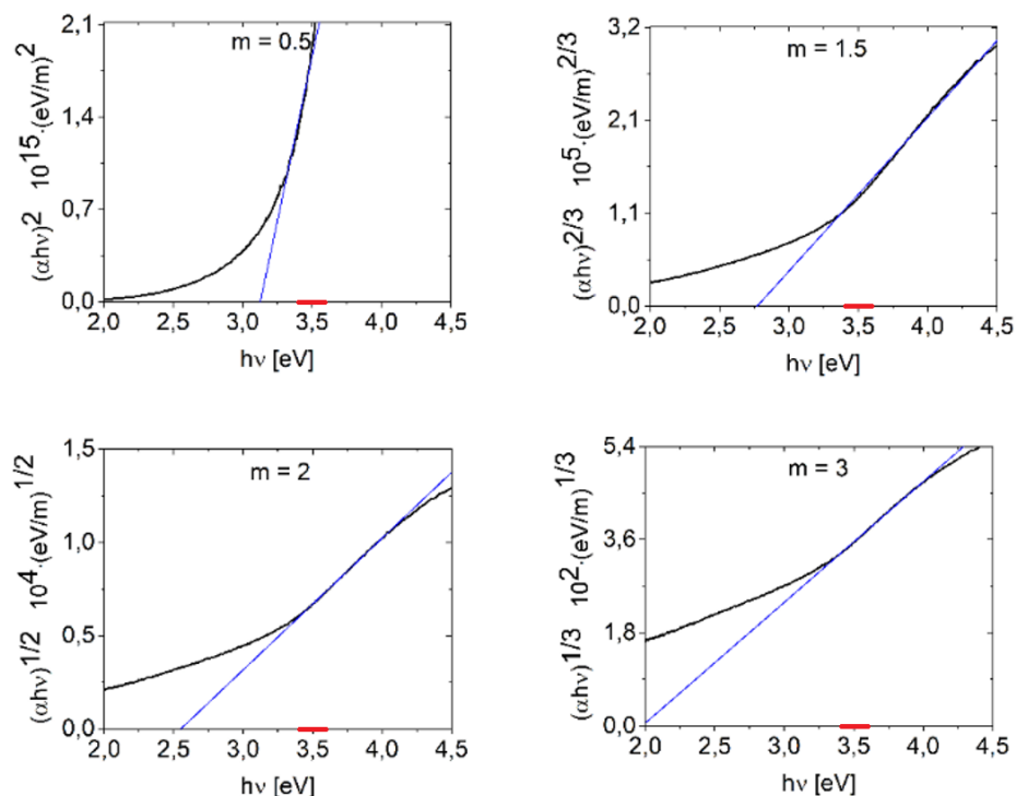
Rysunek 25 Metoda Tauca zastosowana dla próbki \text{TiO}_2 . Dopasowano prostą do każdego z zakładanych parametrów m , w wąskim zakresie energii w pobliżu krawędzi absorpcji (zaznaczonym na osi h\nu kolorem czerwonym).
