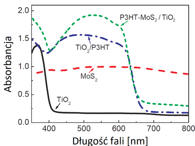
Rysunek 10 Widma absorpcji dla: \text{TiO}_2 , \text{MoS}_2 , \text{TiO}_2 / P3HT oraz P3HT - \text{MoS}_2 / \text{TiO}_2 94 .
