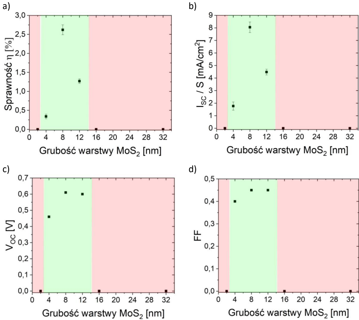
Rysunek 59 a) Sprawność \eta , b) gęstość prądu zwarcia \frac{I_{sc}}{S} ,
