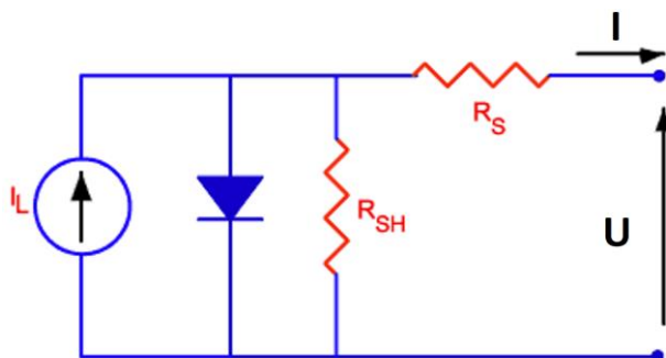
Rysunek 23 Schemat obwodu ogniwa słonecznego z uwzględnieniem rezystancji szeregowej R_s oraz równoległej R_{sh} 116 .
