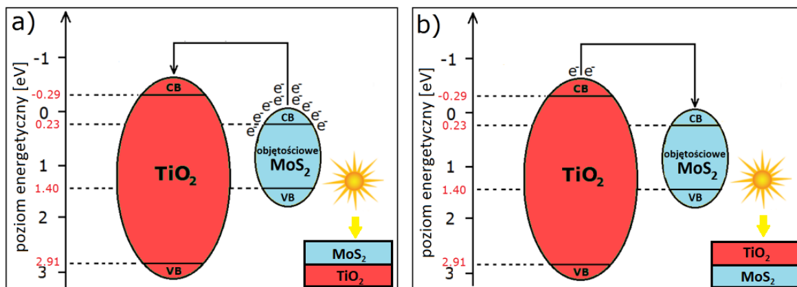
Rysunek 7 Diagram poziomów energetycznych oraz transportu elektronów
