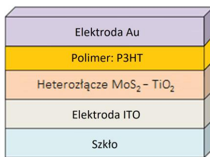
Rysunek 17 Schemat układu wielowarstwowego tworzący ogniwo słoneczne na bazie heterozłączy \text{MoS}_2 - \text{TiO}_2 , gdzie heterozłącze może być zarówno planarne jak i objętościowe (Rysunek 14).
