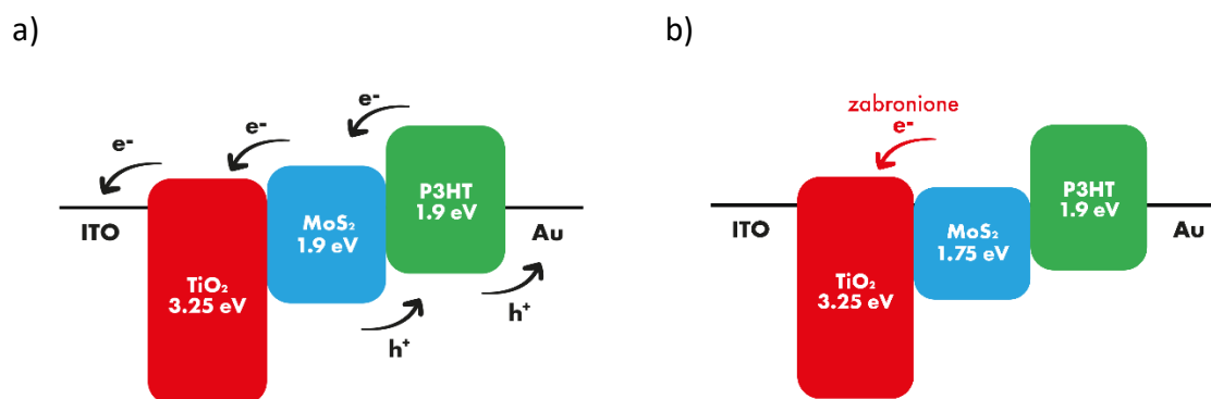
Rysunek 62 Poziomy energetyczny układ materiałów wchodzących w skład ogniwa na bazie polimeru P3HT, MoS 2 oraz TiO 2 ; z szerokością przerwy energetycznej MoS 2 wynoszącą a) 1,9 eV oraz b) 1,75 eV; e - oznacza elektron, h + oznacza dziurę.
