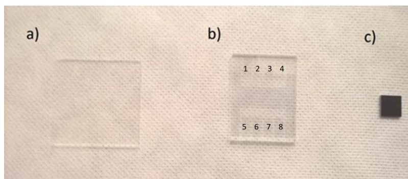
Rysunek 16 Zdjęcie przykładowych podłoży użytych w procesie nanoszenia cienkich warstw: a) kwarcowe, b) podłoże szklane wraz z elektrodami ITO (numery 1 – 8 wskazują na kolejne elektrody), c) krzemowe.
