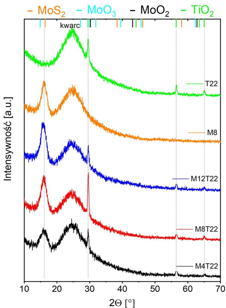
Rysunek 38 Dyfraktogramy heterozłączy planarnych \text{MoS}_2/\text{TiO}_2 oraz próbek referencyjnych M8 i T22. Użyto nazw skróconych, np. M4T22 oznacza próbkę zawierającą \text{MoS}_2 : 4 nm / \text{TiO}_2 : 22 nm.
