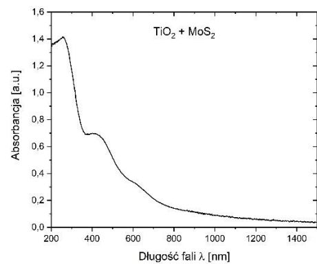
Rysunek 30 Widma absorpcji promieniowania świetlnego UV - ViS dla wygrzewanego
