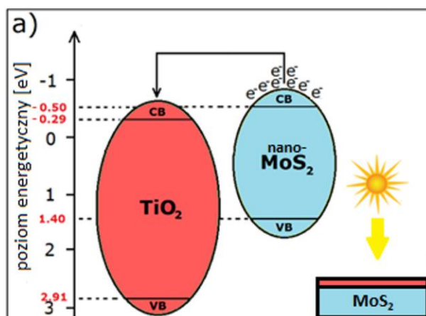
Rysunek 9 Diagram poziomów energetycznych oraz transportu elektronów w heterozłączu planarnym \text{MoS}_2 / \text{TiO}_2 względem normalnej elektrody wodorowej NHE w przypadku słabej absorpcji \text{TiO}_2 oraz zajścia rozmiarowego efektu kwantowego w \text{MoS}_2 . Czerwonym kolorem przedstawiono cienką warstwę \text{TiO}_2 .
