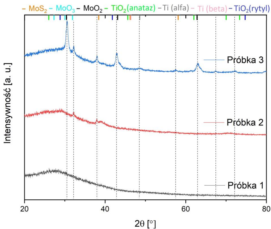
Rysunek 18 Dyfraktogramy próbek powstałych w wyniku rozpylania magnetonowego przy użyciu katod \text{MoS}_2 oraz \text{Ti} w atmosferze \text{O}_2 .
