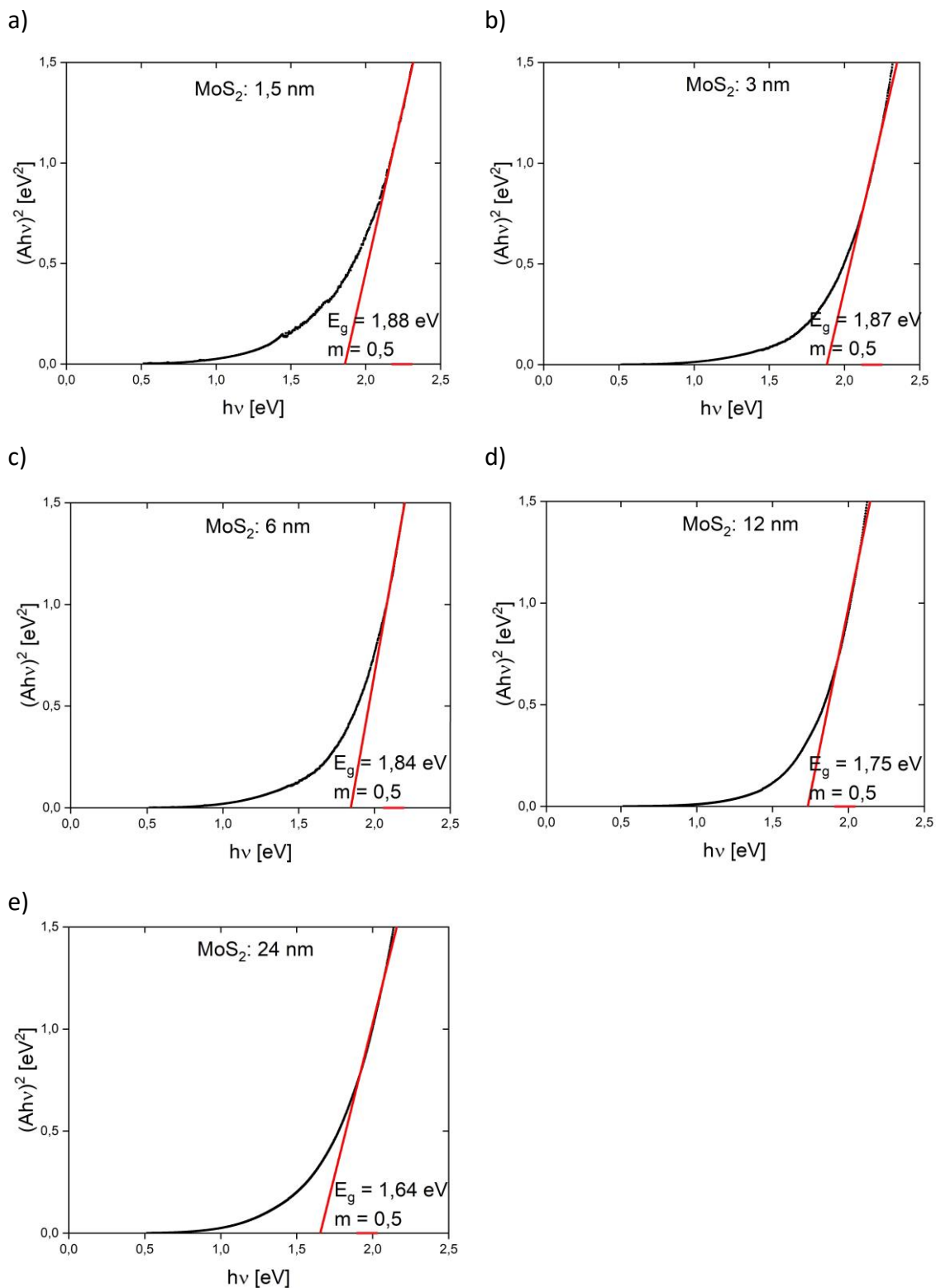
Rysunek 49 Analiza metodą Tauc widm absorpcji cienkich warstw MoS 2 o grubościach:
