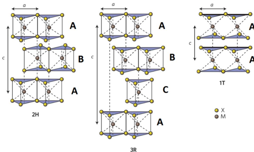
Rysunek 5 Trzy główne odmiany krystaliczne MoS 2 (M - atom molibdenu, X - atom siarki) 84 .
