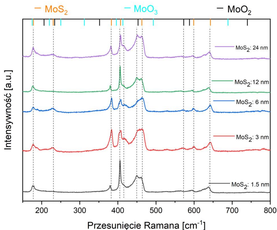
Rysunek 31 Widmo Ramana dla cienkich warstw \text{MoS}_2 różniących się grubością (od 1.5 nm do 24 nm) dla rezonansowej linii lasera o długości fali 633 nm.
