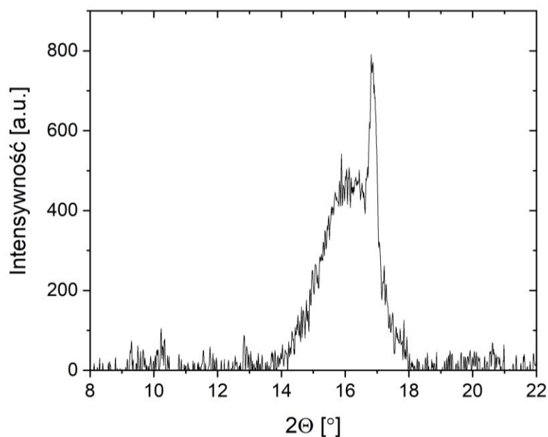
Rysunek 45 Dyfraktogram cienkiej warstwy MoS 2 wykonany rok po wytworzeniu próbki.
