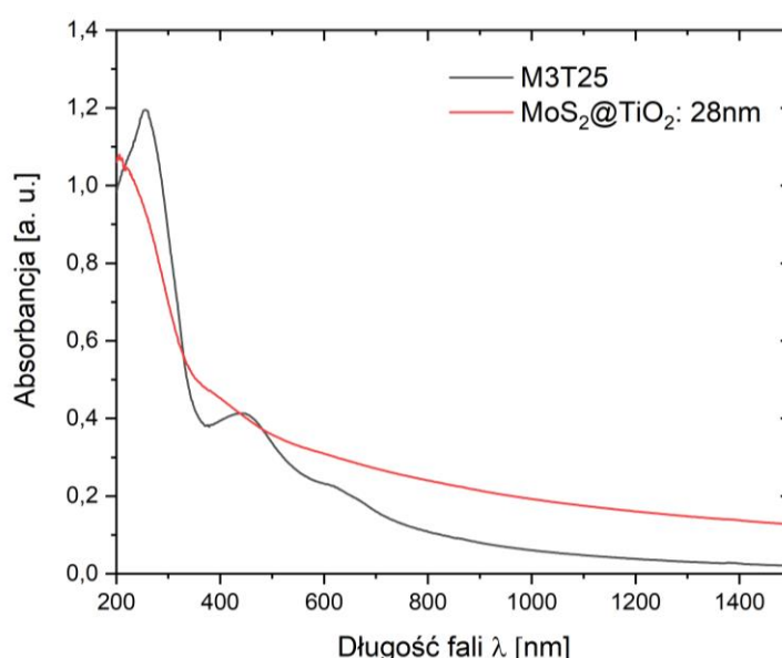
Rysunek 65 Widma absorpcji promieniowania światelnego UV - ViS dla heterozłączy M3T25 oraz \text{MoS}_2@\text{TiO}_2 : 28 nm zarejestrowane w temperaturze pokojowej.
