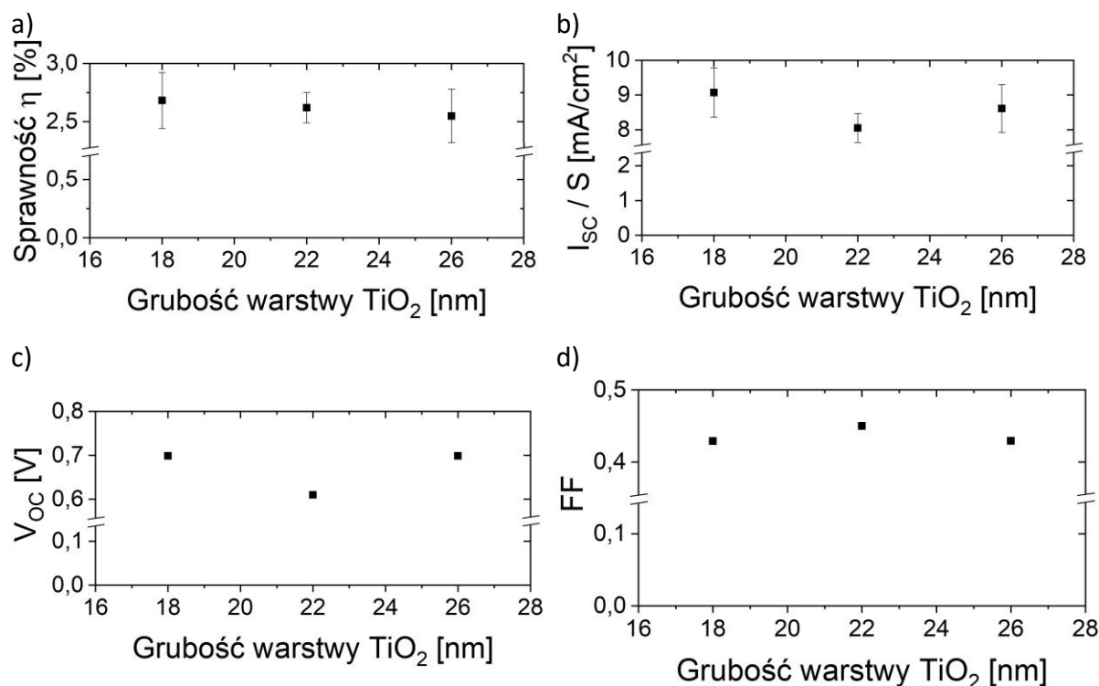
Rysunek 60 a) Sprawność \eta , b) gęstość prądu zwarcia \frac{I_{sc}}{S} , c) napięcie ogniwa otwartego nieobciążonego V_{oc} oraz d) współczynnik wypełnienia „fill factor” FF w funkcji grubości warstwy TiO 2 dla ogniw M8T18, M8T22 oraz M8T26 opartych na heterozłączach planarnych MoS 2 / TiO 2 (spoza serii).
