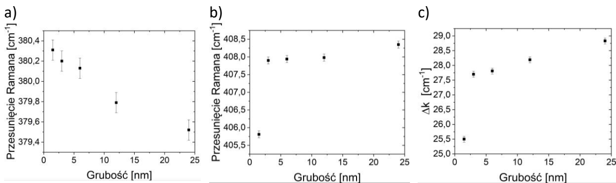
Rysunek 56 Przesunięcia pików głównych modów \text{MoS}_2 : E_{2g} (a) oraz A_{1g} (b) w zależności od grubości warstwy \text{MoS}_2 ; (c) zależność pomiędzy różnicą \Delta k pomiędzy przesunięciami Ramana głównych pików odpowiadającym modom A_{1g} oraz E_{2g} , a grubością warstwy.
