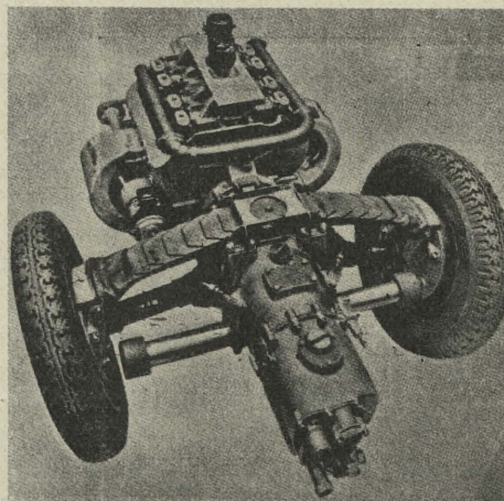
Rys. 3. Zwarty blok napędowy samochodu „Tatra” 77.
