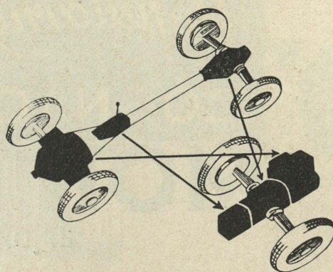
Rys. 1. Zamiast organów napędu rozmieszczonych na całej długości pojazdu, jeden zwarty blok napędowy.
