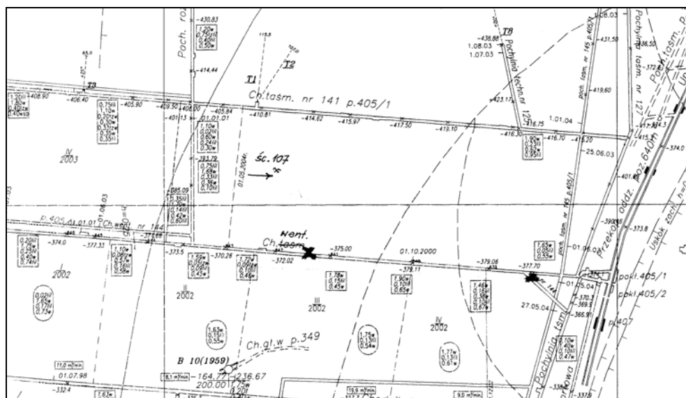
Rys. 5. Rejon badań w chodniku wentylacyjnym i pochylni taśmowej ściany 107 w pokładzie 405/1 w KWK „Brzeszcze”
