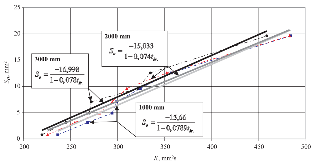
Rys. 3. Charakterystyka sondy areometrycznej — S_o = f(K)
