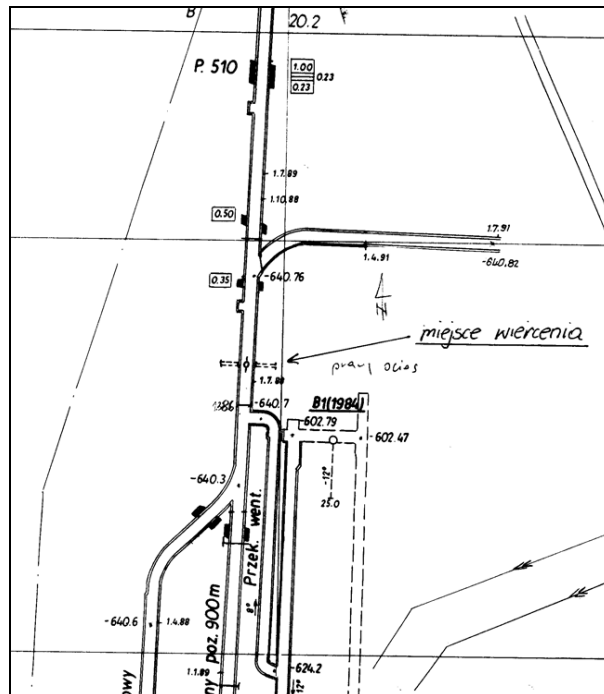
Rys. 4. Rejon badań w przekopie głównym poz. 900 m w KWK „Brzeszcze”
