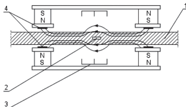
Rys. 4. Rozkład pola magnetycznego w uszkodzonej linie [6]
