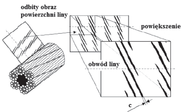
Rys. 2. Pomiar wielkości starć drutów metodą in print odbicia powierzchni liny [8]
