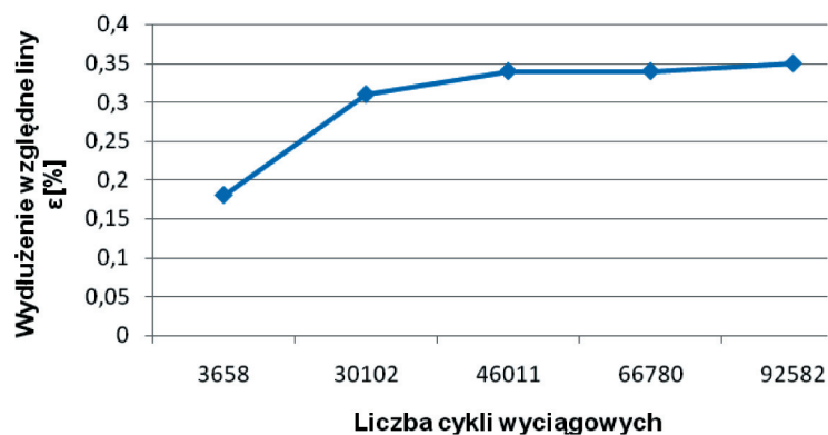
Rys. 13. Wykres wydluzenia względnego liny \varepsilon w funkcji liczby cykli wyciągowych, lina wschodnia, zestaw 5
