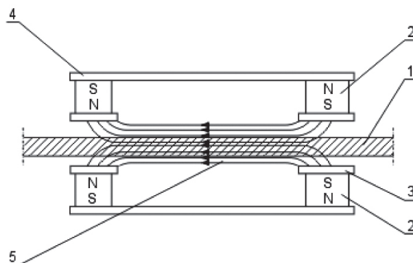
Rys. 3. Rozkład linii pola magnetycznego w nieuszkodzonej linie [6]
