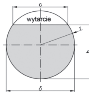
Rys. 1. Obliczanie powierzchni starcia drutu [8]
