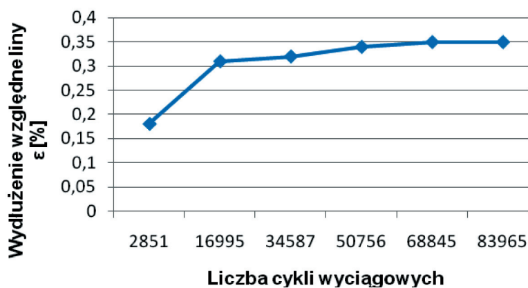
Rys. 11. Wykres wydluzenia względnego liny \varepsilon w funkcji liczby cykli wyciągowych, lina wschodnia, zestaw 4
