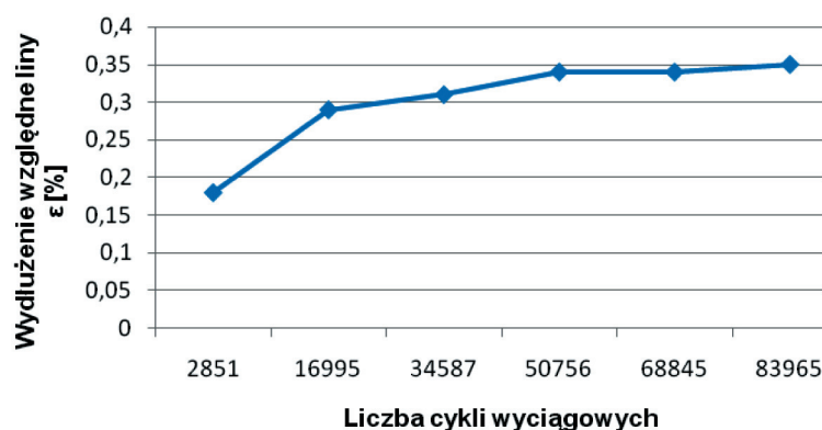
Rys. 12. Wykres wydluzenia względnego liny \varepsilon w funkcji liczby cykli wyciągowych, lina zachodnia, zestaw 4
