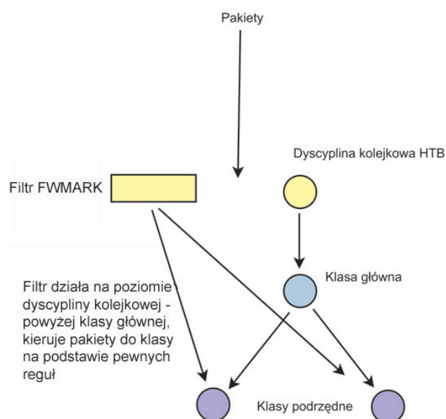
Rys. 2. Reguły współdziałania filtra klasyfikującego FWMARK z dyscypliną kolejkową HTB
