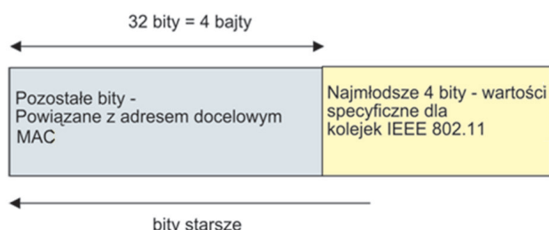
Rys. 5. Format pola MARK w schemacie mieszanym
