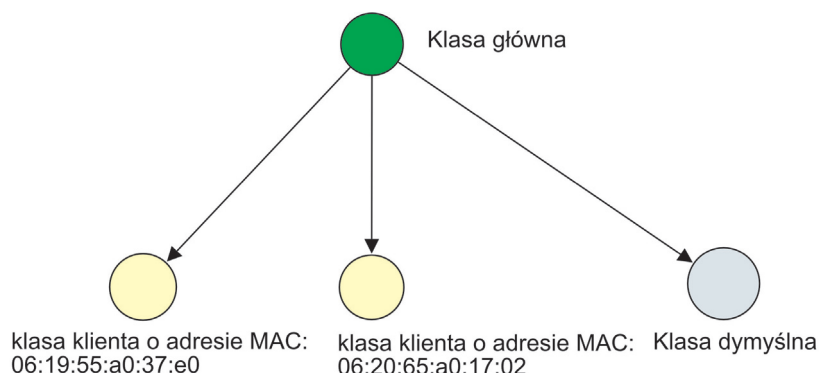
Rys. 3. Hierarchia klas dyscypliny kolejkowej HTB
