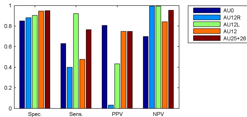
Rysunek C.5: Konfiguracja 3, klasyfikator kNN
