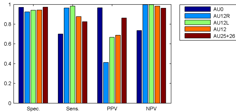
Rysunek C.4: Konfiguracja 2, klasyfikator QDA
