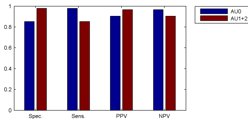
Rysunek C.14: Rozpoznawanie kształtów — test 2, klasyfikator kNN
