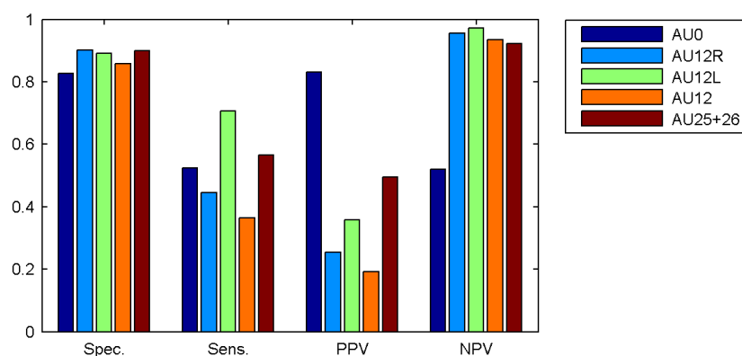
Rysunek C.7: Konfiguracja 4, klasyfikator kNN
