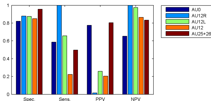
Rysunek C.6: Konfiguracja 3, klasyfikator QDA
