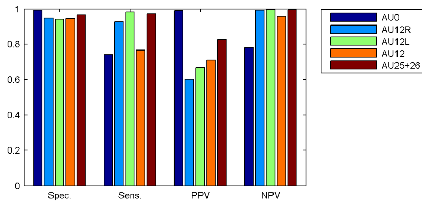
Rysunek C.2: Konfiguracja 1, klasyfikator QDA
