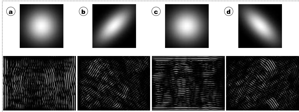
Rysunek 6.4: Maski filtrów Gabora i odpowiadające im obrazy po filtracji. Parametry: f_G = 0.125 , (a) \theta_G = 0^\circ , (b) \theta_G = 45^\circ , (c) \theta_G = 90^\circ , (d) \theta_G = 135^\circ
