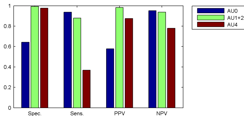
Rysunek C.19: Rozpoznawanie kształtów — test 4, klasyfikator LDA
