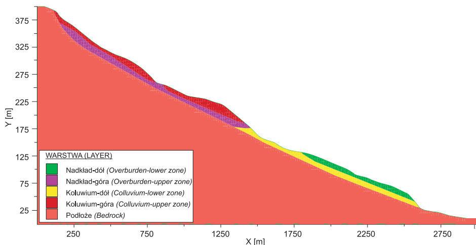
Fig. 4. Podział modelu numerycznego na warstwy (strefy) geotechniczne
