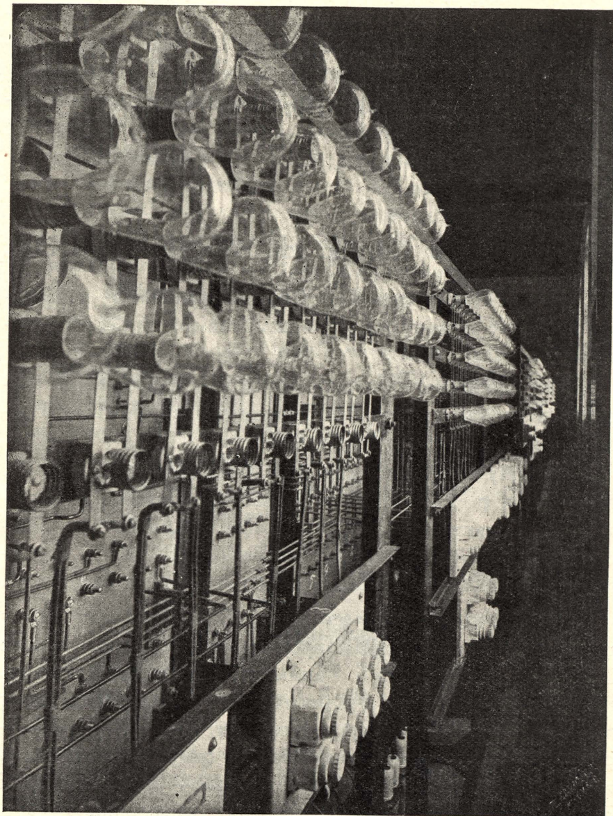
STACJA ROZDZIELCZA W HALI MASZYN KATEDRY ELEKTROTECHNIKI.
