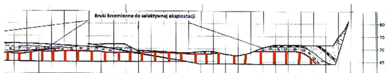
Rys. 1. Fragment kartowania geologicznego skarpy V poziomu P/Szczerców
