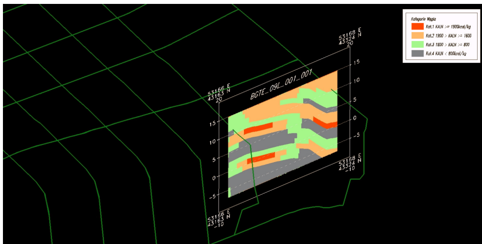
Rys. 9. Przekrój przez stratamodel
