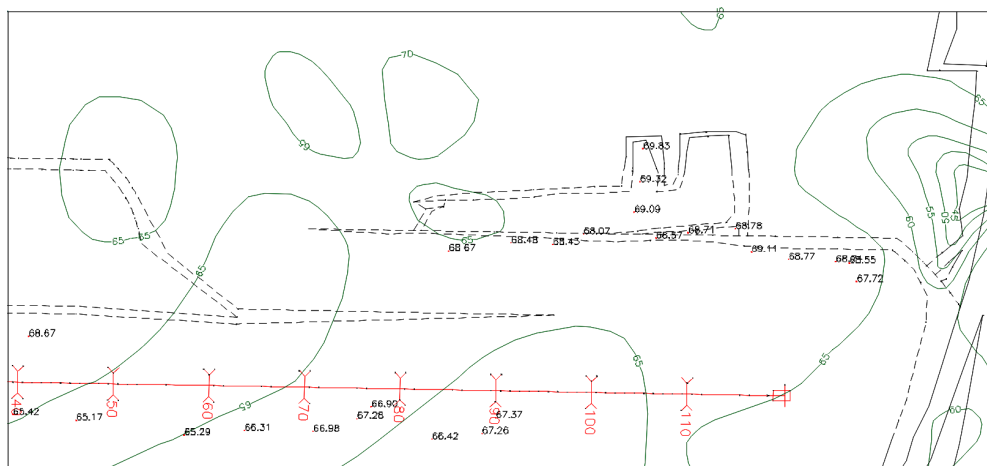
Rys. 2. Fragment mapy stropu węgla z naniesionymi zamierzeniami GPS stropu węgla; w tle referencja mapy sztygarskiej
