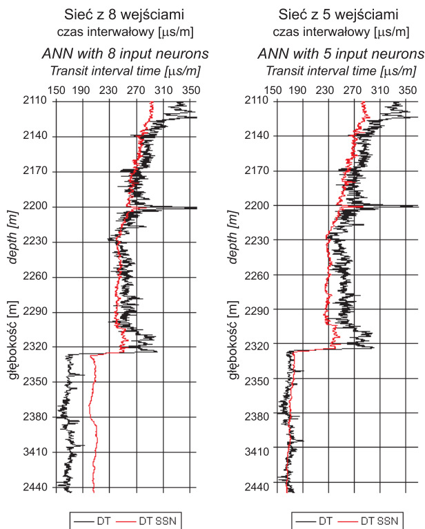
Fig. 3. Porównanie wyników pracy perceptronów z 8 i 5 neuronami na wejściu w otworze W4
