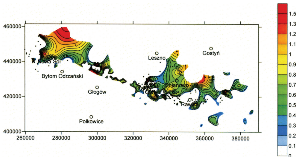
Rys. 4. Zdolność magazynowa złoża Na1 w środkowej części monokliny przedśudeckiej
