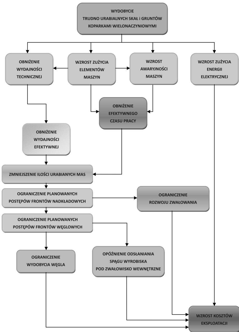
Rys. 3. Schemat wpływu występowania trudno urabialnego nadkładu na efekty eksploatacyjne
