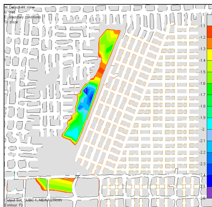
Rys. 15. Współczynniki bezpieczeństwa dla filarów w polu G-12/7 dla wariantu 2 (kolor szary dla obszarów calizny, likwidacji lub dla filarów upodatnionych)
