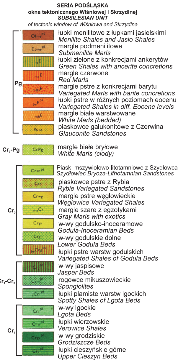
Fig. 3. Przykład zastosowania profilowań ciągłych w rejonie Raciechowice – Stadniki: I – mapa geologiczna (wg Burtan 1954, 1974), II – przekrój geologiczny wzdłuż linii A–B, III – przekrój geoelektryczny z interpretacją geologiczną
