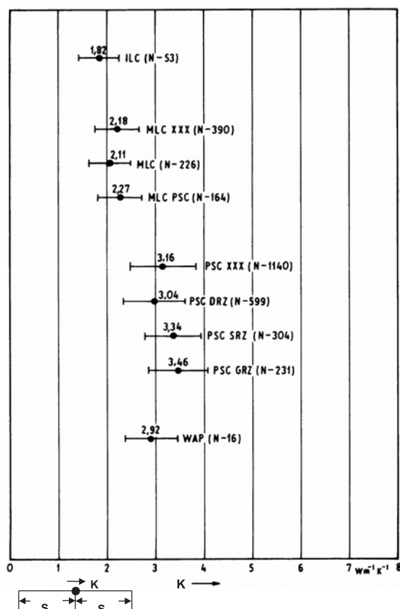
Fig. 7. Statystyczna charakterystyka przewodności cieplnej w utworach karbonu GZW – kierunek badania równoległy do osi otworu: ILC – ilowce; MLC – mułowce (MLC XXX – mułowce ogółem, MLC PSC – mułowce piaszczyste); PSC – piaskowce (PSC XXX – piaskowce ogółem, PSC DRZ – piaskowce drobnoziarniste, PSC SRZ – piaskowce średnioziarniste, PSC GRZ – piaskowce gruboziarniste); WAP – wapienie, K – średnia arytmetyczna przewodności cieplnej, S – odchylenie standardowe, N – liczba pomiarów
