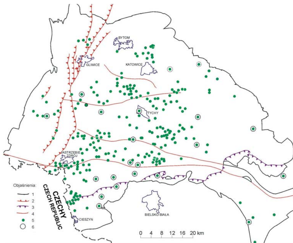
Fig. 1. Mapa lokalizacji otworów z pomiarami temperatury w obszarze GZW: 1 – wychodnie utworów karbonu węglonośnego na stropie paleozoiku, 2 – nasunięcia, 3 – północny zasięg fliszu karpackiego, 4 – uskoki, 5 – otwory, w których wykonano ciągle pomiary temperatury, 6 – otwory, w których wykonano pomiary własności cieplnych. Elementy budowy geologicznej przyjęto wg Buła & Kotasa red. (1994)
