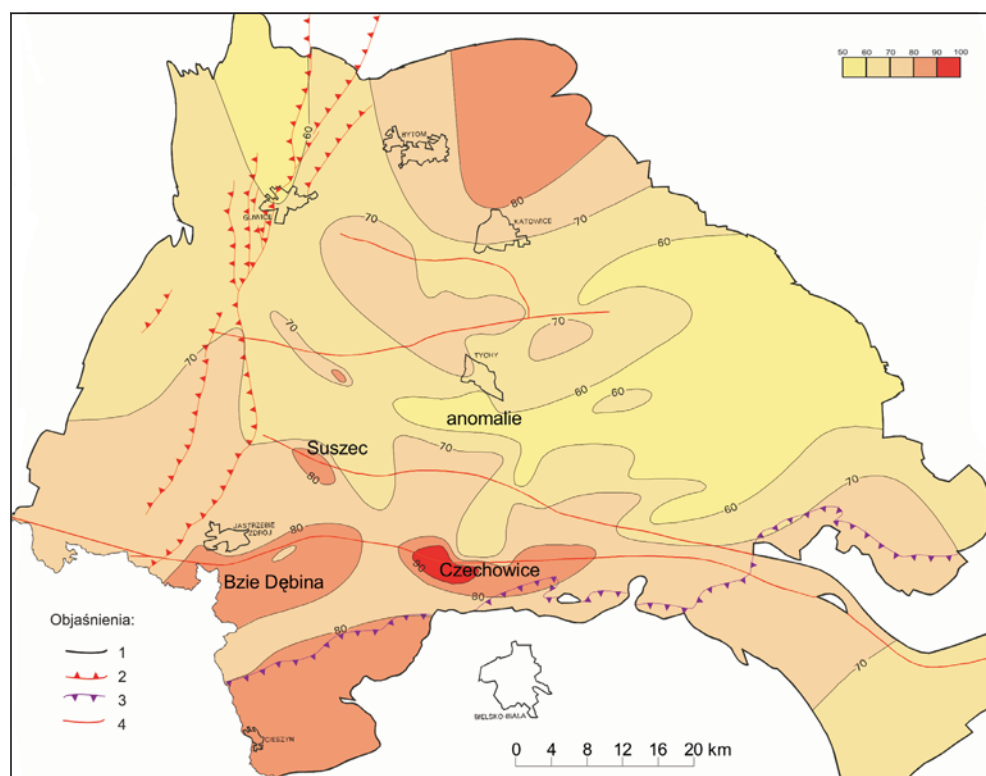
Fig. 10. Mapa gęstości strumienia ciepłego na obszarze GZW [ \text{mW/m}^2 ]: 1 – wychodnie utworów karbonu węglonośnego na stropie paleozoiku, 2 – nasunięcia, 3 – północny zasięg fliszu karpacciego, 4 – uskoki. Elementy budowy geologicznej przyjęto wg Buły & Kotasa red. (1994)
