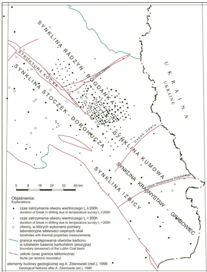
Fig. 2. Lokalizacja otworów, w których wykonano pomiary geotermiczne w obszarze LZW
