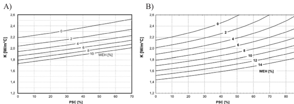
Fig. 8. Wykres zależności współczynnika przewodności efektywnej skał K [ \text{W/m}^\circ\text{C} ] od zawartości piaskowców: A) LZW; B) GZW
