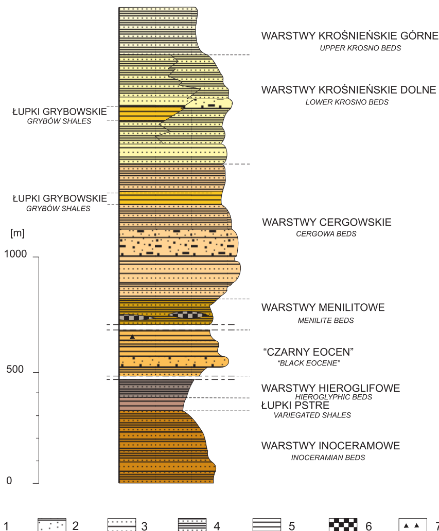
Fig. 4. Profil litostratigraficzny jednostki dukielskiej w oknie tektonicznym Mszany Dolnej (Burtan et al. 1992, zmienione): 1 – piaskowce zlepieńcowate, 2 – gruboławicowe piaskowce, 3 – piaskowce średnio- i cienkoławicowe z łupkami, 4 – łupki z cienkoławicowymi piaskowcami, 5 – łupki mułowcowe i ilaste, 6 – rogowce, 7 – syderyty
