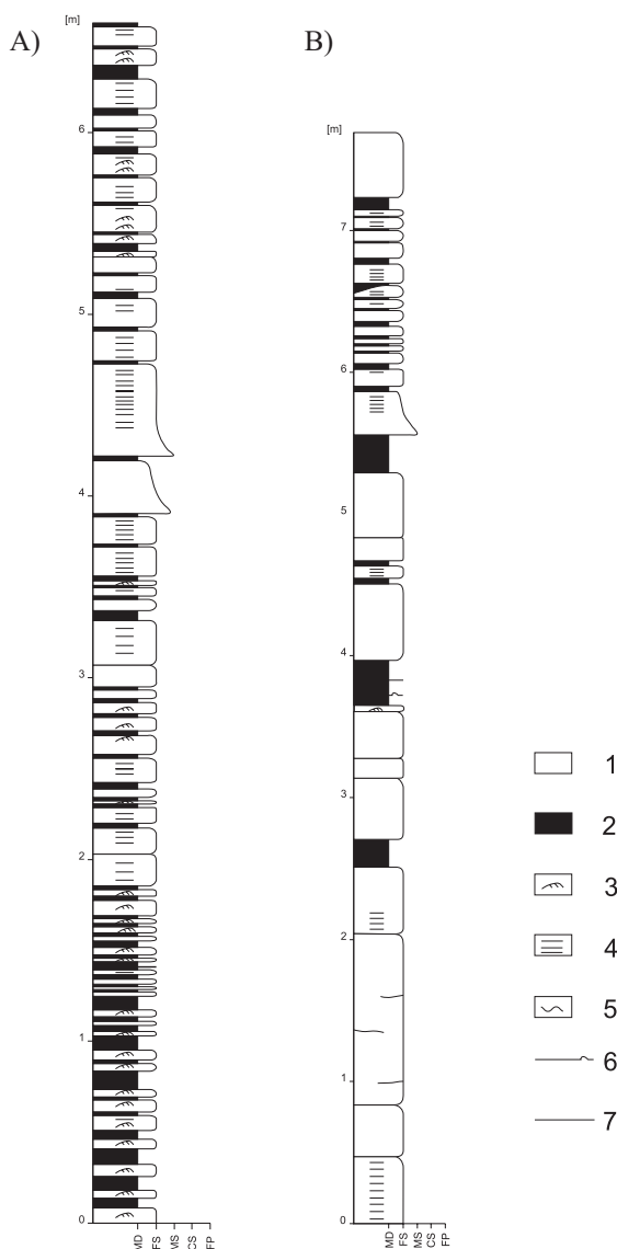
Fig. 6. Profile osadów lobowych: A) profil D20 Mszana Górna, przysiółek Węglarze; B) profil P2 Podobin, przysiółek Rąpty: 1 – piaskowce, 2 – łupki mułowcowe i ilaste, 3 – warstwowanie przekątne, 4 – laminacja równoległa, 5 – laminacja falista, 6 – cienkie piaskowce (poniżej 3 cm) riplemarkowe, 7 – cienkie piaskowce (poniżej 3 cm) laminowane i masywne; frakcje: MD – iłowa i pyłowa, FS – piasek drobny, MS – piasek średni, CS – piasek gruby, FP – żwir drobny
