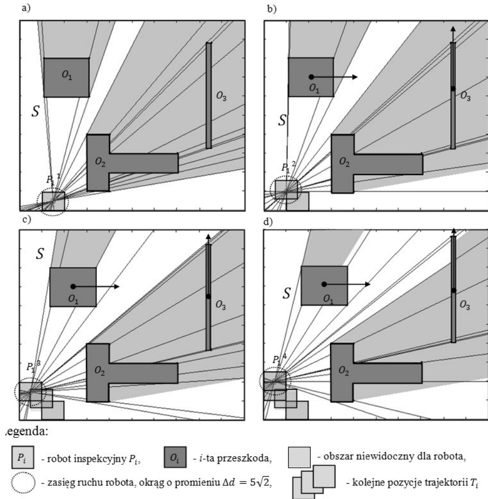
Rys. 2. Pozycje robota inspekcyjnego otrzymywane z algorytmu
