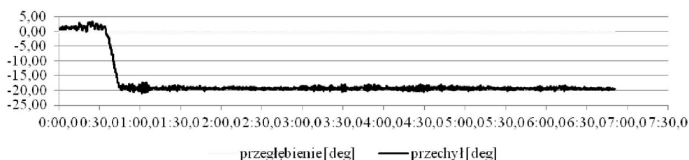
Rys. 3. Przykład przebiegu czasowego kolysań bocznych kątowych statku (roll)
