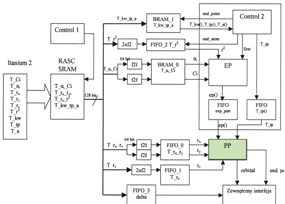
Rys. 4. Osadzenie jednostki PP w strukturze modułu Orbital
