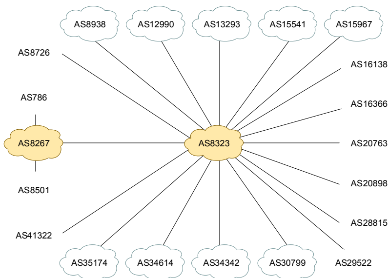
Rys. 11. Połączenia systemów autonomicznych Cyfronetu i ich sąsiadów
