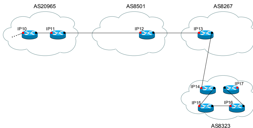
Rys. 14. Struktura połączeń na poziomie IR oraz AS dla Cyfronetu
